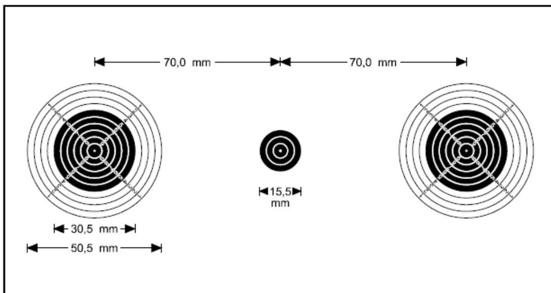
Bersaglio Mobile 10 metri cartaceo
